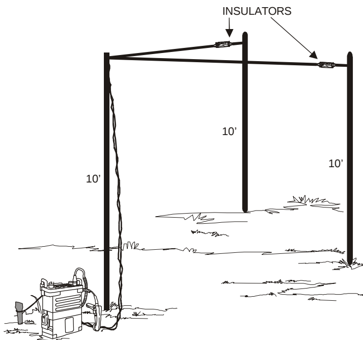
Figure 6-13. Vee Antenna.
