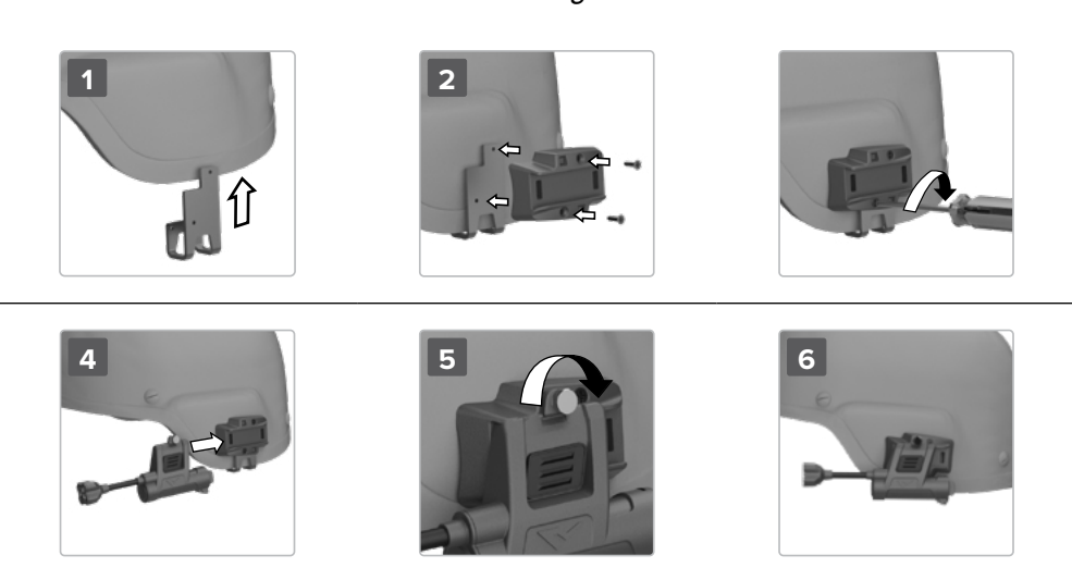
Abbildung 8 – Picatinny-Schienenbefestigung
