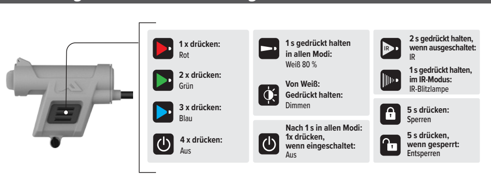
Abbildung 2 – Schalterbedienung
